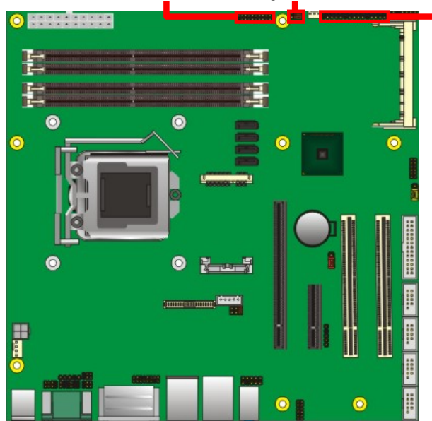
CN_USB1/2
